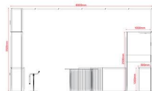
结构施工图 (单位: mm)
